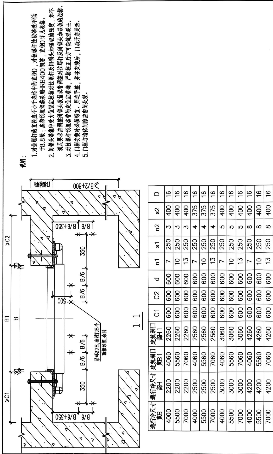
固定门槛双扇密闭门 (二)
